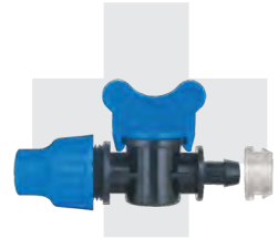
MINİ VANA Kilitli Bağlantı - Grommet D.Ç:18mm MINI VALVE Lock Type - Grommet-(DD:18 mm)
